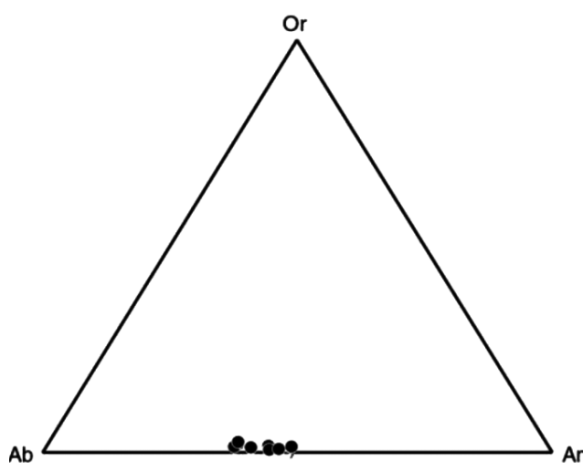
شکل ۲- ترکیب شیمی کانی‌های پلاژیوکلاز در سنگ‌های کوارتز-دیوریت تخت سلیمان.
