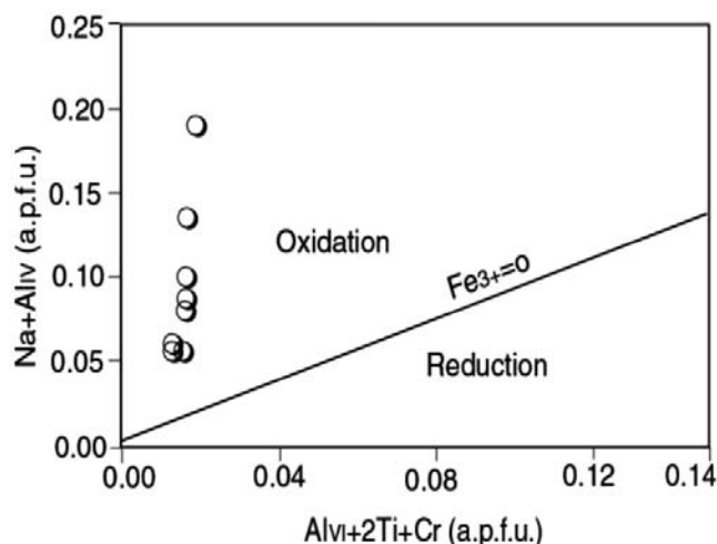
شکل ۵- تعیین فوگاسیته اکسیژن ماگمای اولیه سنگ‌های کوارتز-دیوریت بر اساس ترکیب شیمی کانی‌های کلینوپیروکسن (Schweitzer et al., 1979).
