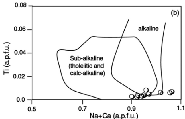
شکل ۶- ویژگی نیمه قلیایی سنگ‌های کوارتز-دیوریت تخت سلیمان (a) نمودار \text{SiO}_2 (wt%) - \text{Al}_2\text{O}_3 (wt%)، مرز جداکننده بین ترکیب ماگماهای قلیایی، نیمه قلیایی و فوق قلیایی بر اساس Le Bas (1962) است. (b) نمودار \text{Ti} (a.p.f.u.) - \text{Na}+\text{Ca} (a.p.f.u.) بر اساس Leterrier et al. (1982).
