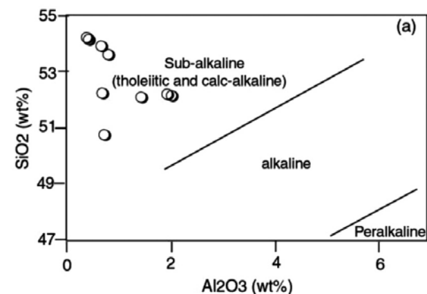
شکل ۶- ویژگی نیمه قلیایی سنگ‌های کوارتز-دیوریت تخت سلیمان (a) نمودار \text{SiO}_2 (wt%) - \text{Al}_2\text{O}_3 (wt%)، مرز جداکننده بین ترکیب ماگماهای قلیایی، نیمه قلیایی و فوق قلیایی بر اساس Le Bas (1962) است. (b) نمودار \text{Ti} (a.p.f.u.) - \text{Na}+\text{Ca} (a.p.f.u.) بر اساس Leterrier et al. (1982).
