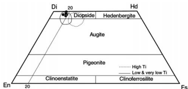
شکل ۴- ترکیب کانی‌های پیروکسن در نمودار En-Fs-Di-Hd (Morimoto et al., 1988).
