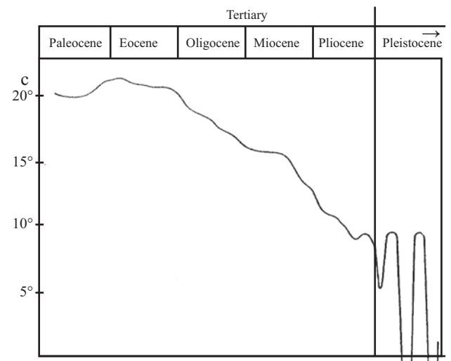
نمودار ۱- نمایش تغییرات آب و هوایی و افت قابل توجه دما در اواخر میوسن و پلیوسن (برگرفته از Tachmuller, 1975).
