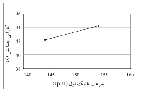
شکل ۱۲- تأثیر سرعت غلتک اول بر کارایی عملیاتی
