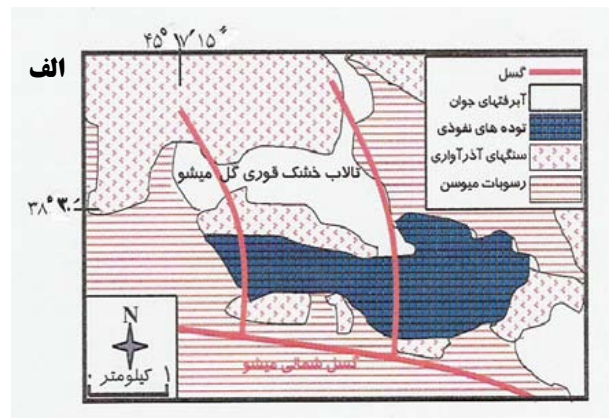
شکل ۸- الف) نقشه موقعیت و ویژگیهای زمین شناسی آبگیر خشک میشو (برگرفته از نقشه زمین شناسی به مقیاس ۱:۱۰۰۰۰۰ تسوج و قره ضیاء الدین با تغییرات)، ب) یادگانه رودخانه‌ای ایجاد شده در بستر آبگیر خشک میشو
